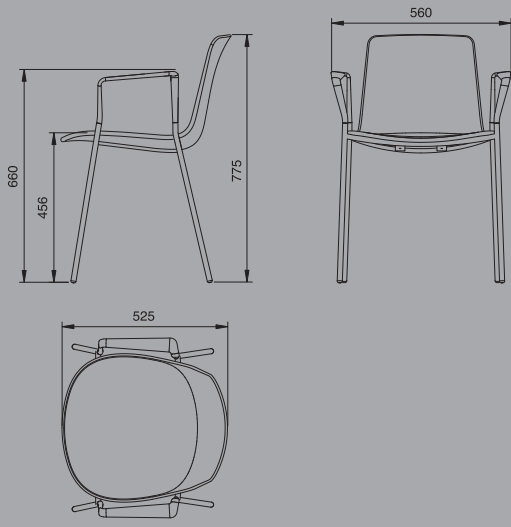
LOTTUS CON BRAZOS DE ALUMINIO WITH ALUMINIUM ARMRESTS
